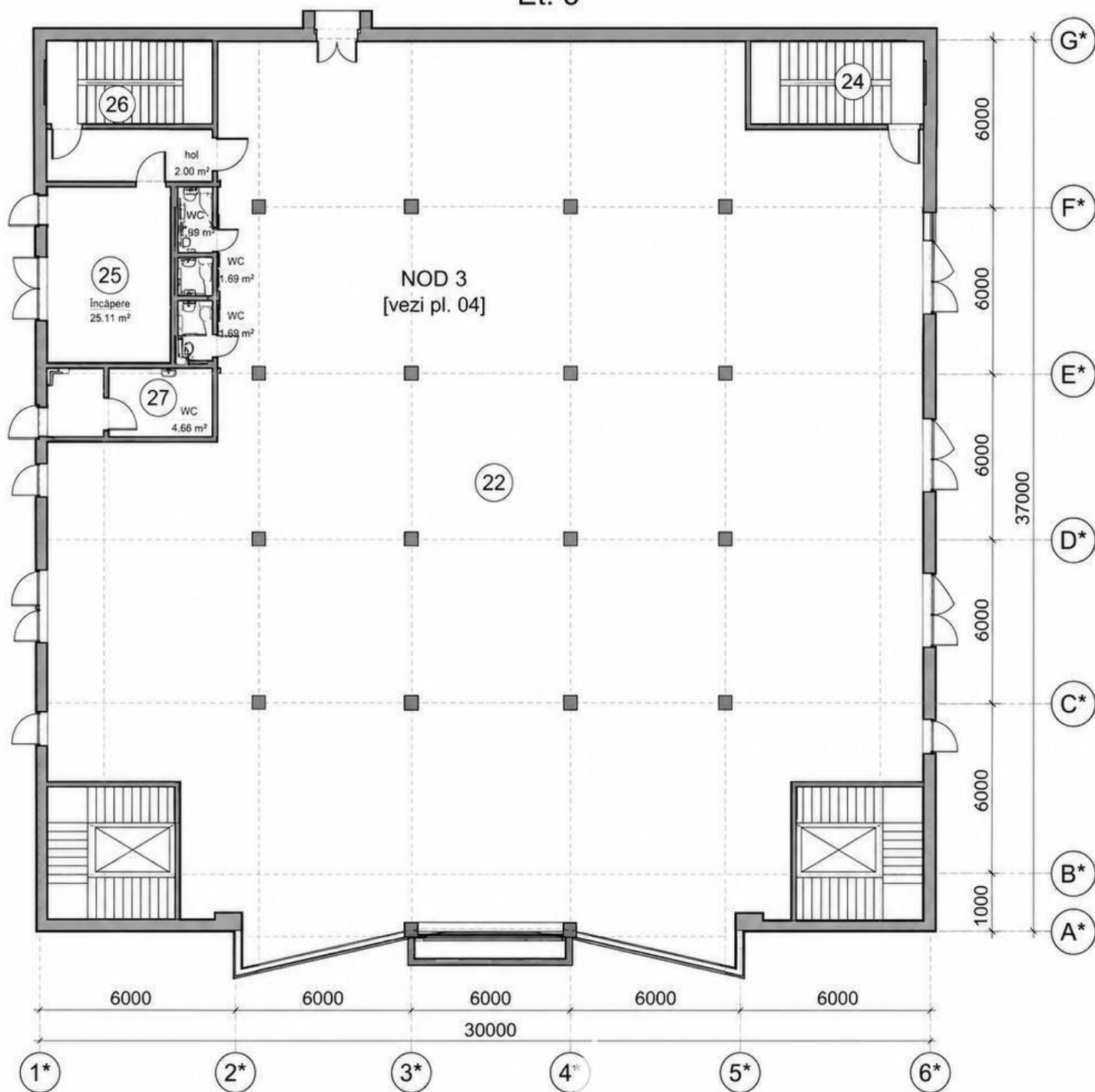
Specificația încăperilor etaj cotă +8,900
